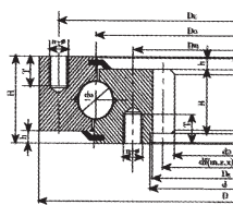
Серия QN, тип B
