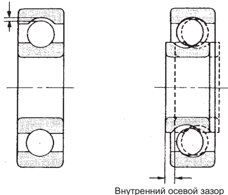
Рис 5.1. Внутренний зазор
