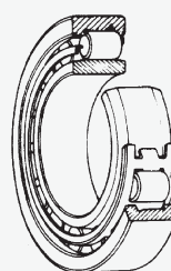
Роликовый цилиндрический подшипник Рис. 1.3
