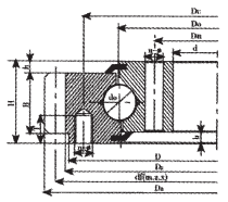
Серия QW, тип C
