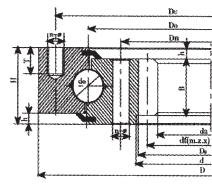
Серия QN, тип C
