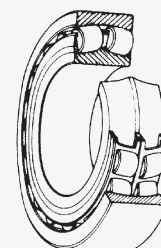
Роликовый сферический подшипник Рис. 1.6
