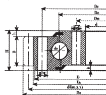
Серия QW, тип A
