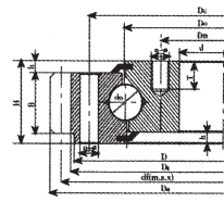
Серия QW, тип D
