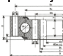
Серия QN, тип A
