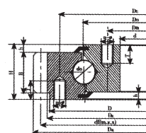
Серия QW, тип B
