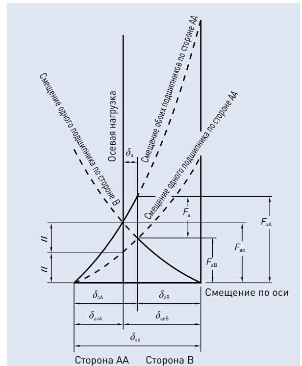
Рис. 4.6 Смещение по оси компоновки DBD с преднатягом
