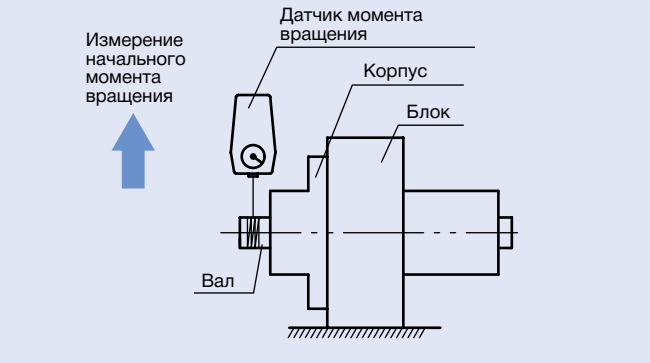
Рис. 1.23 Метод начального момента вращения
