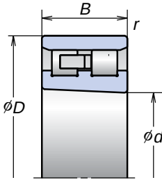
NN39 Коническое внутреннее отверстие
