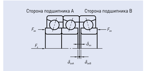
Рис. 4.5 Компоновка DBD с преднатягом
