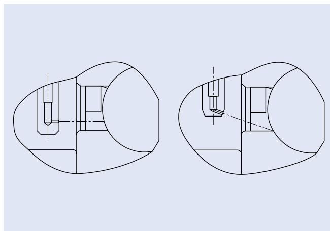
Рис. 9.1 Угол насадки
