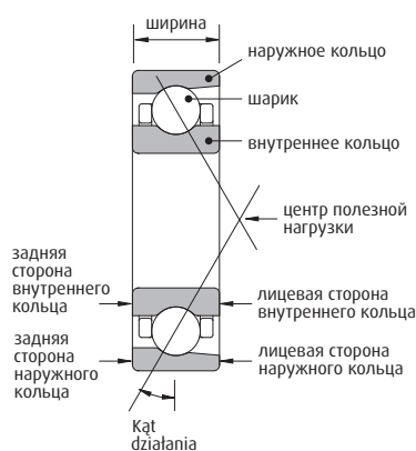
Однорядный радиально-упорный шарикоподшипник
