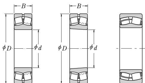
Цилиндрическое отверстие
