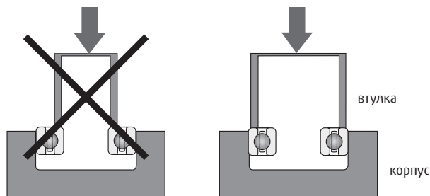
Установка подшипника в корпус
