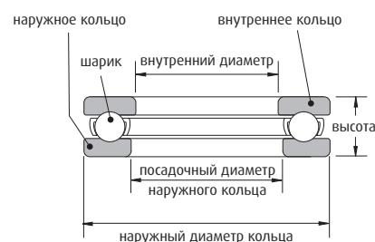
Одинарный упорный шарикоподшипник
