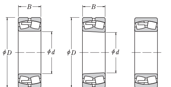
Цилиндрическое отверстие
