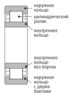
Цилиндрический роликоподшипник (тип NU)
