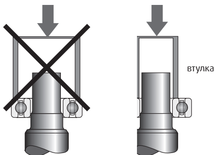
Установка подшипника на вал
