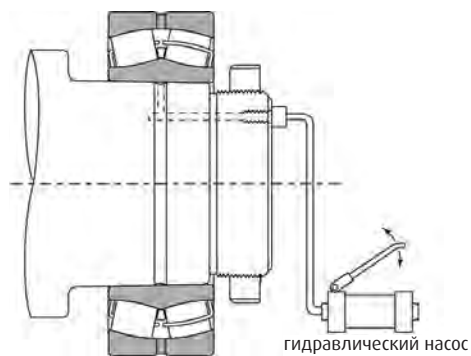
Извлечение при помощи впрыскивания масла
