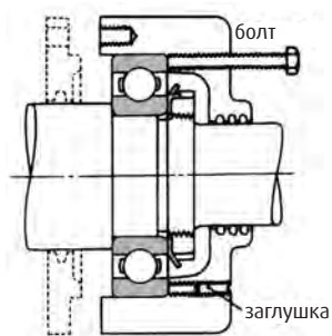
Извлечение наружного кольца при помощи демонтирующих болтов
