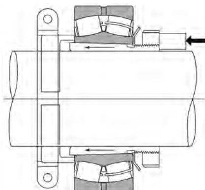
Извлечение втулки при помощи осевого давления с остановками
