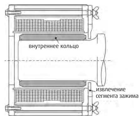
Извлечение внутреннего кольца при помощи индукционного нагревателя
