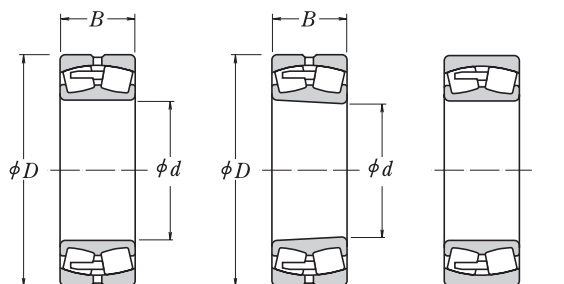
Цилиндрическое отверстие
