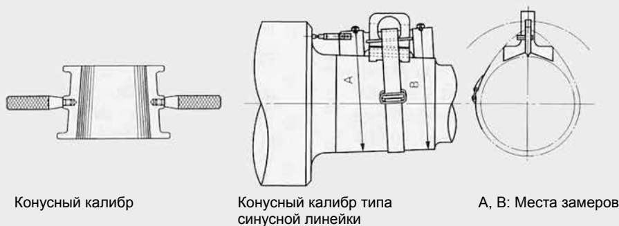
Рис. 8.2 Конический вал
