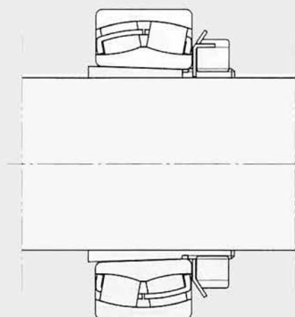
Рис. 1.12 Цилиндрический вал, стопорная шайба (закрепительная втулка)
