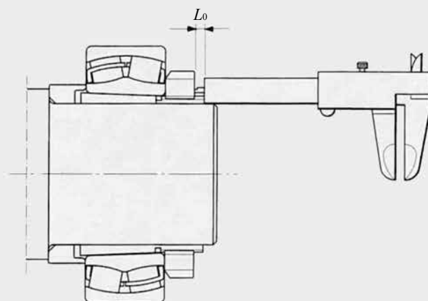
Рис. 2.14 Измерение штангенциркулем
