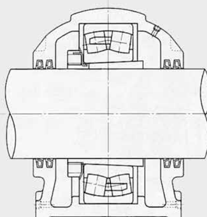
Рис. 1.17 Свободный край
