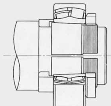
Рис. 2.9 Регулировка зазора
