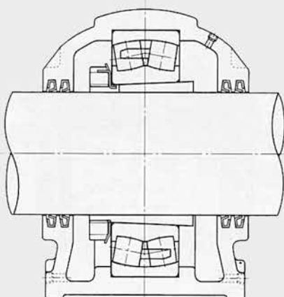
Рис. 1.16 Закрепленный край
