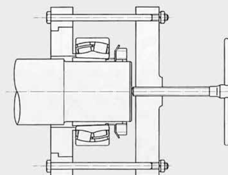
(б) Вариант с закрепительной втулкой
