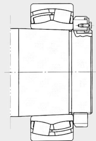
Рис. 1.10 Конический вал, стопорный бугель
