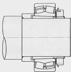
Рис. 6.11 Вид в собранном состоянии
