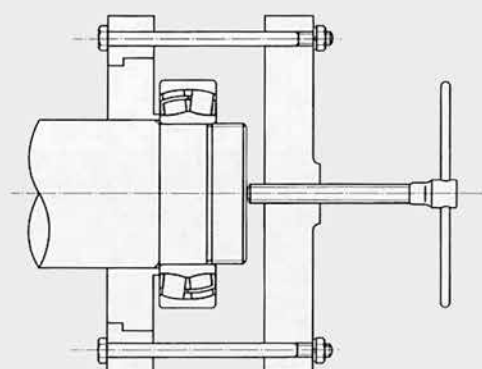
(а) Вариант цилиндрического вала
