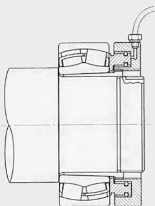
Рис. 7.7 Способ применения гидравлической гайки
