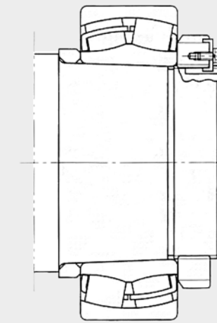
Рис. 1.11 Конический вал, стопорный бугель (с дистанционным кольцом)
