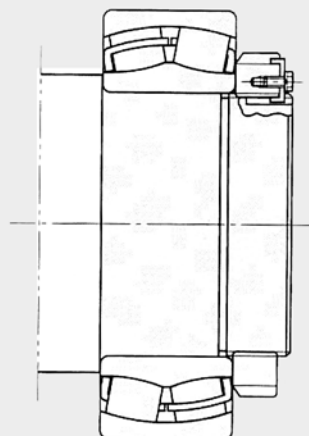
Рис. 1.7 Цилиндрический вал, стопорный бугель
