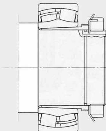
Рис. 1.14 Цилиндрический вал, стопорная шайба (стяжная втулка)
