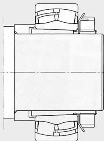
Рис. 1.13 Цилиндрический вал, стопорная шайба (закрепительная втулка с дистанционным кольцом)
