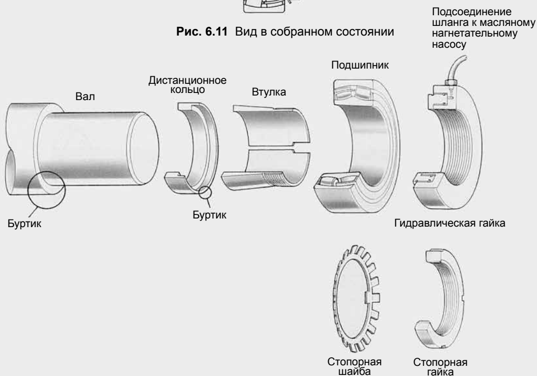
Рис. 6.12 Способ гидравлической гайки
