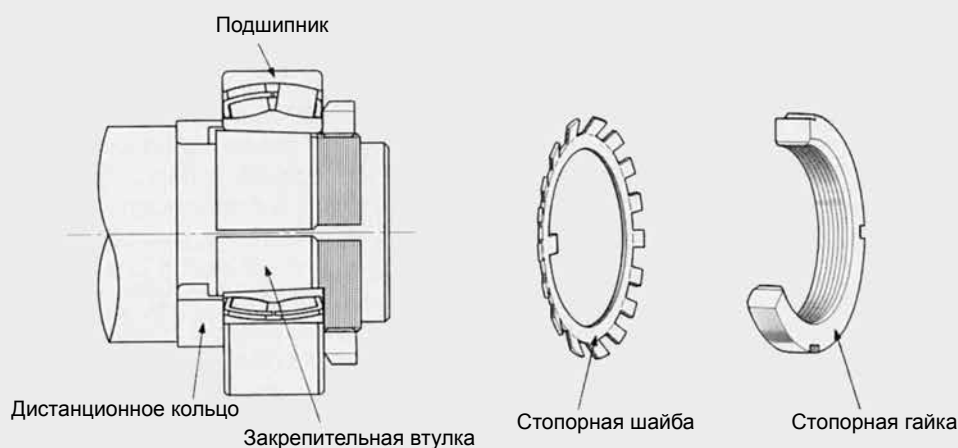
Рис. 2.10 Установка стопорной шайбы по окончании регулировки зазора.
