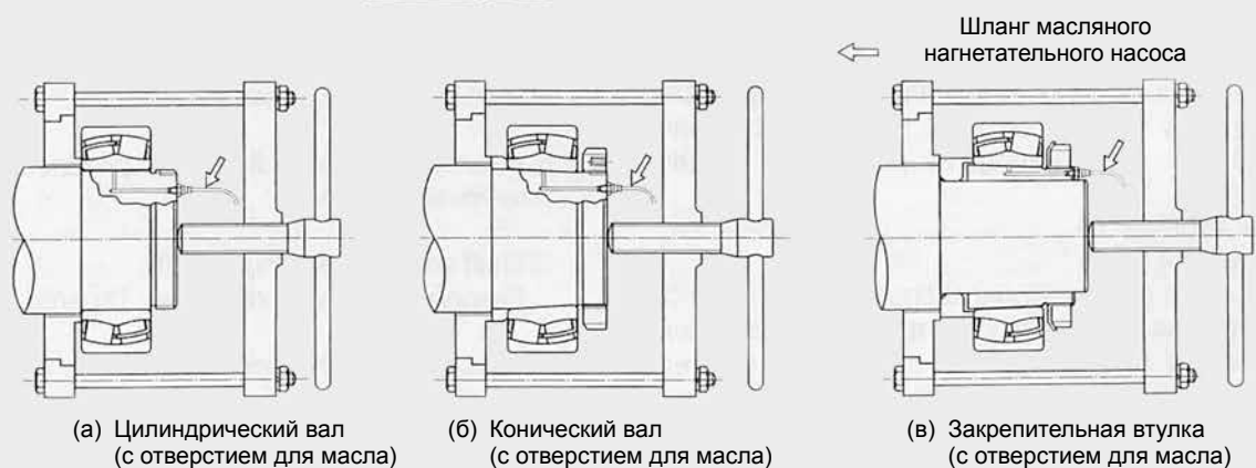
Рис. 7.8 Способ ввода масла под давлением
