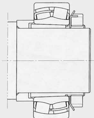
Рис. 2.8 Вид в собранном положении
