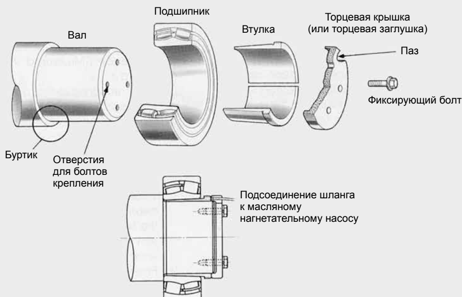
Рис. 6.20 Способ ввода масла под давлением
