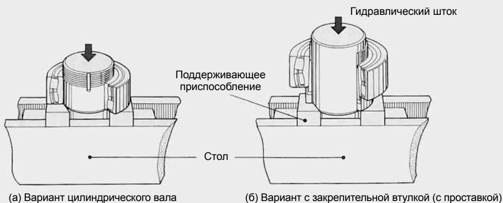
Рис. 7.6 Способ прессования
