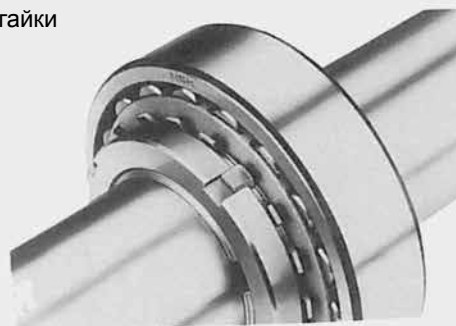
Рис. 2.7 Загибание усов стопорной шайбы
