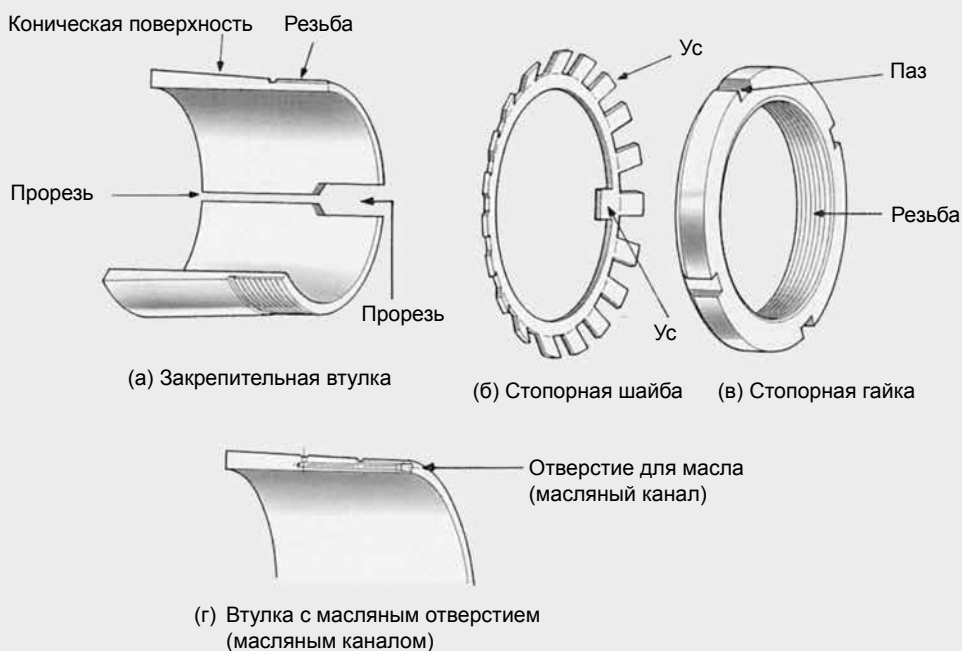
Рис. 2.3 Компоненты закрепительной втулки
