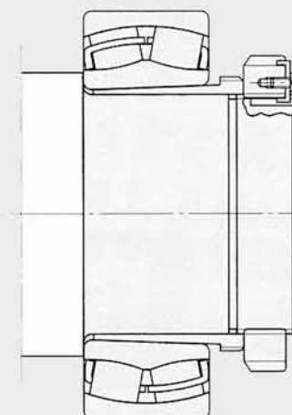
Рис. 1.15 Цилиндрический вал, стопорный бугель (стяжная втулка)
