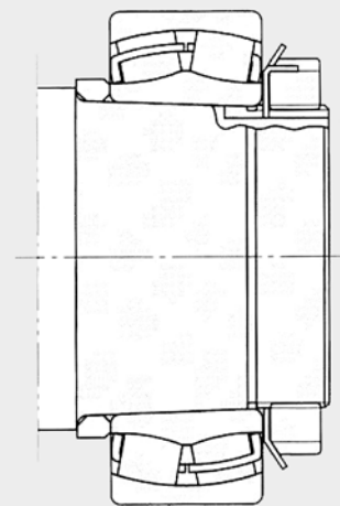
Рис. 1.9 Конический вал, стопорная шайба (с дистанционным кольцом)
