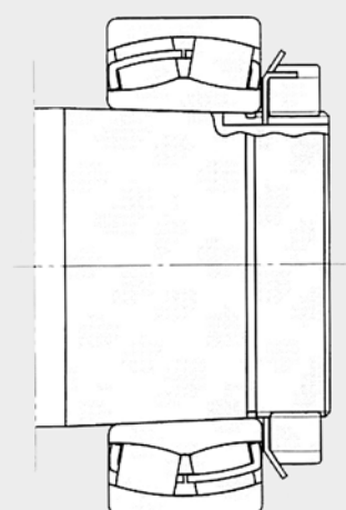
Рис. 1.8 Конический вал, стопорная шайба
