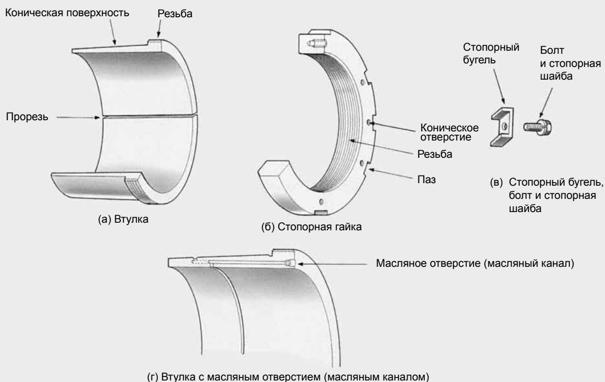
Рис. 2.4 Стяжная втулка
