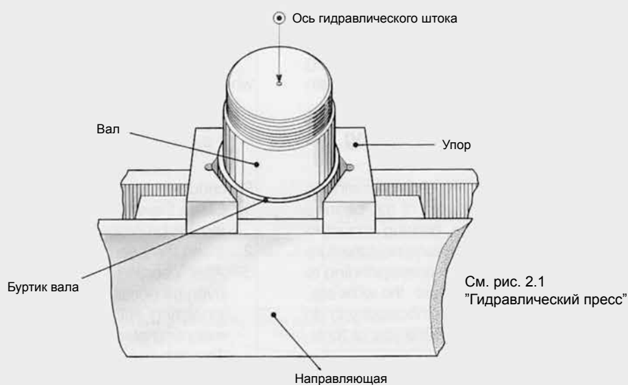
Рис. 6.2 Способ прессования (фиксация вала на столе пресса)
