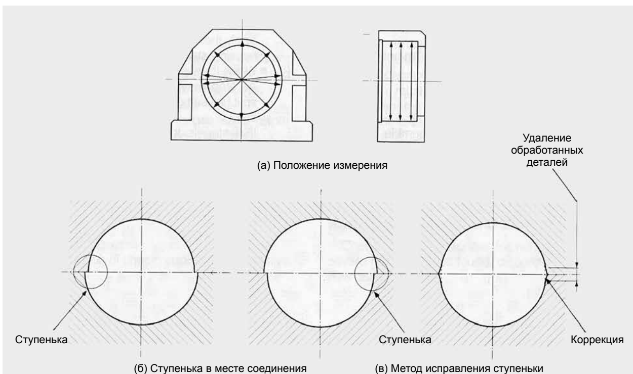
Рис. 8.4 Разрезной корпус
