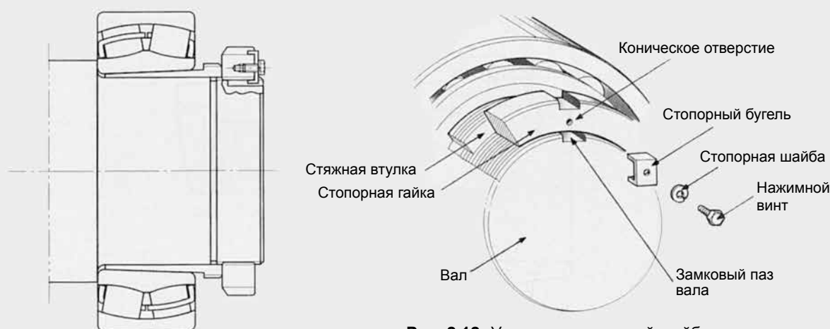
Рис. 2.11 Вид в собранном состоянии
