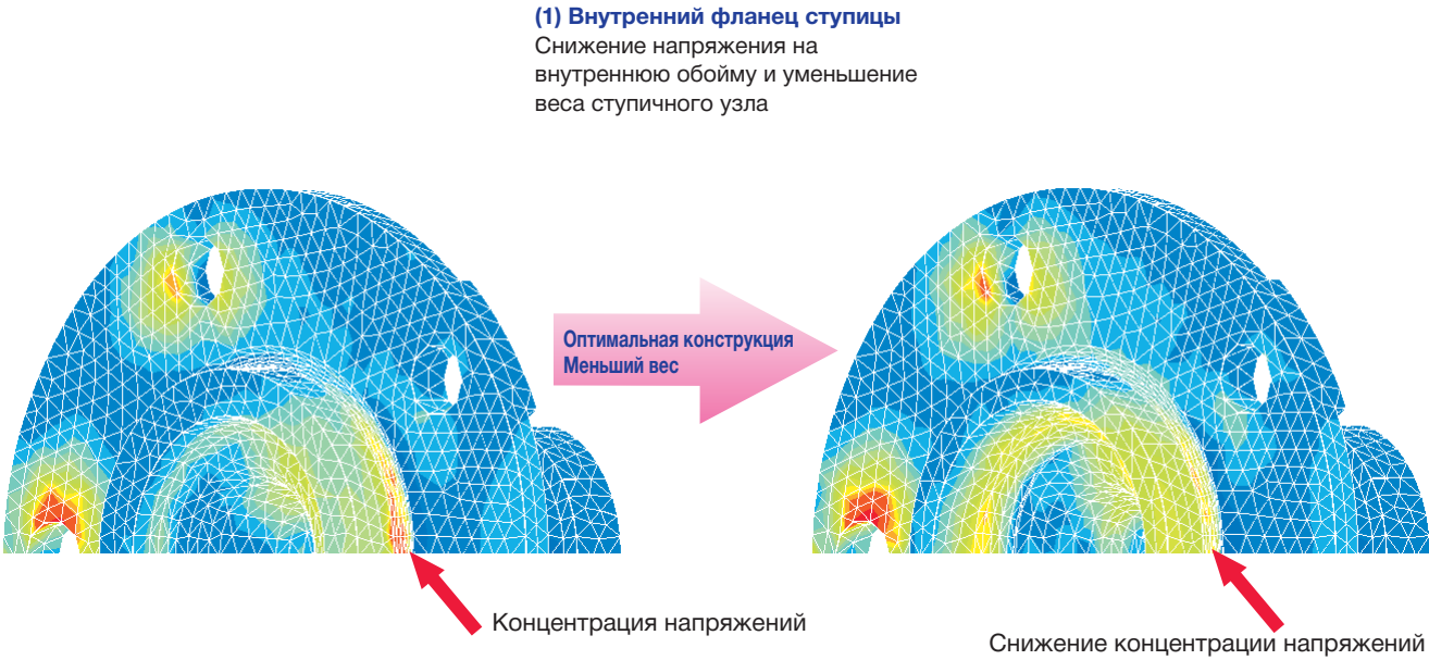
Рис.5. Пример АМКЭ (Внутренний фланец)
