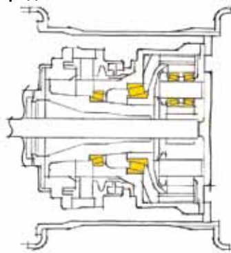
Передний мост
