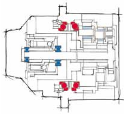
Редуктор
