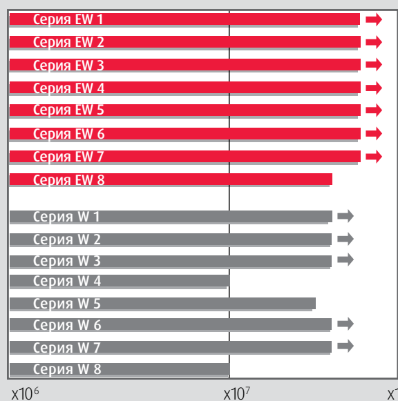
Результаты испытаний прочности сепараторов
