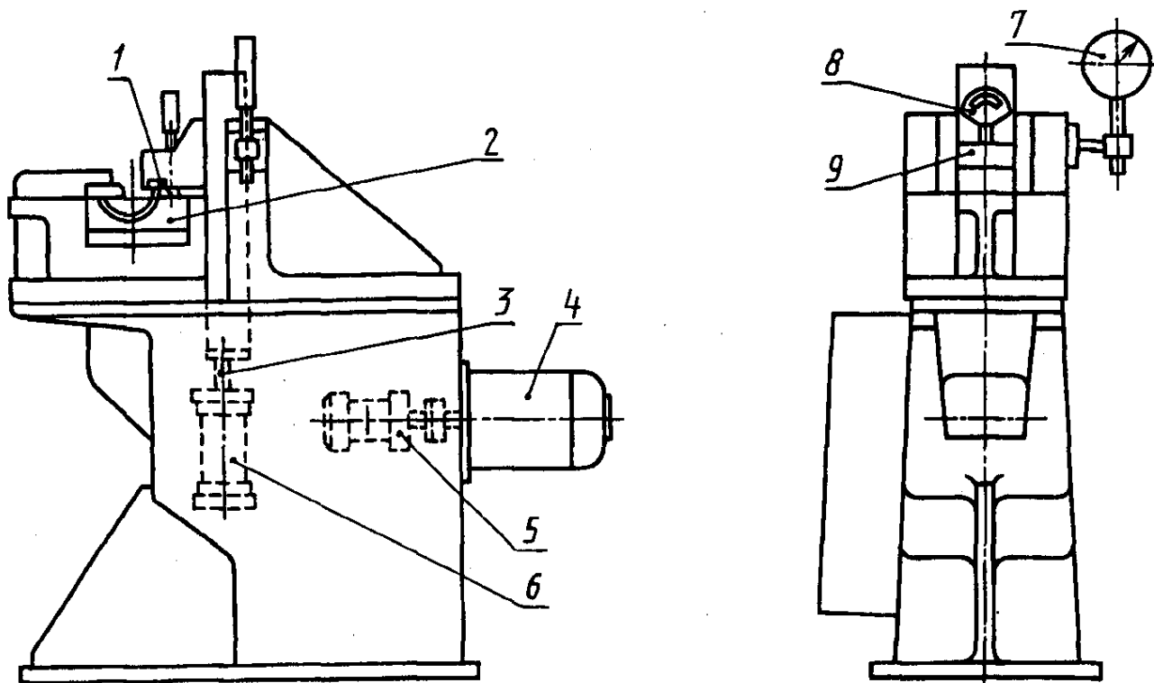
1 — самоустанавливающаяся опорная пята; 2 — контрольный блок; 3 — клапан регулирования давления; 4 — приводной двигатель; 5 — масляный насос; 6 — рабочий цилиндр; 7 — манометр; 8 — индикатор; 9 — подвижная измерительная головка
