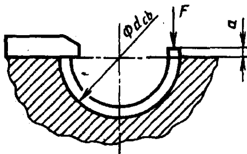
Рисунок 1 — Выступание a
