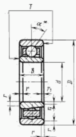
Типы 76000, 36000K7, 36000K, 46000K, 66000K
