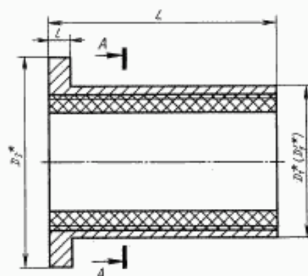
Подшипник типа II
