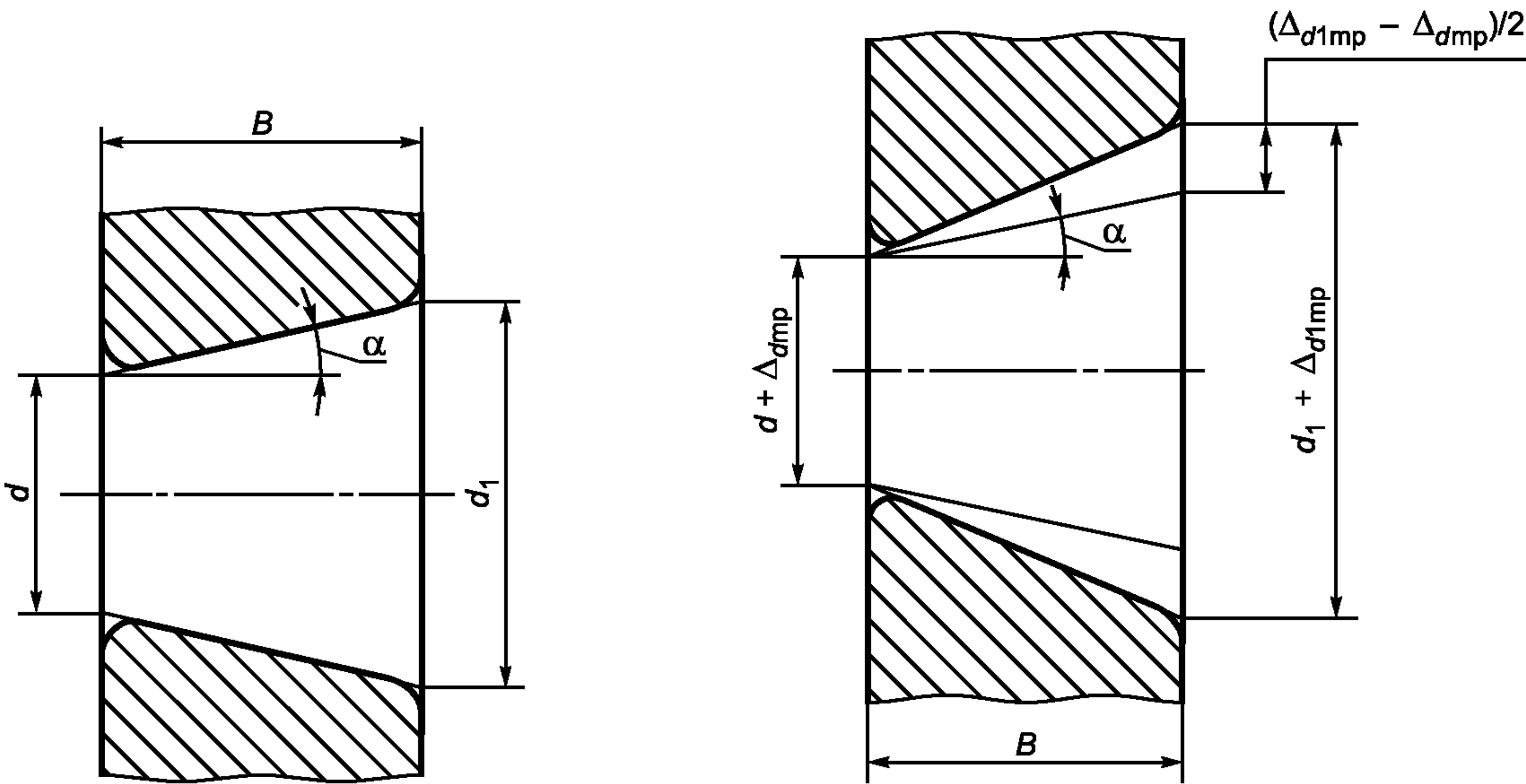
Рисунок 4 — Номинальное коническое отверстие Рисунок 5 — Действительное коническое отверстие
