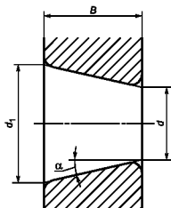
Рисунок 4 — Номинальное коническое отверстие
