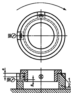
1 — опорный торец упорного борта; 2 — кольцеобразная шлицевая опора; а — предел зоны измерения (таблица 57)
